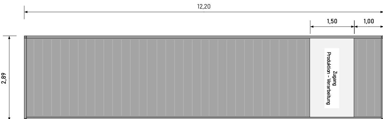
Ansicht D – Seitenansicht mit Übergang zu Produktion
